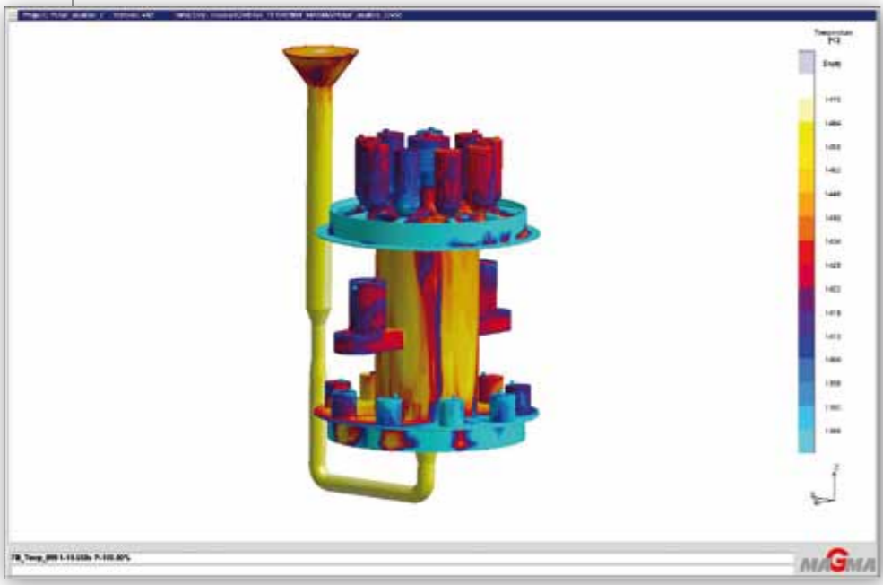
Simulación llenado y solidificación de un tambor de cable Cable drum mould filling and solidification simulation
